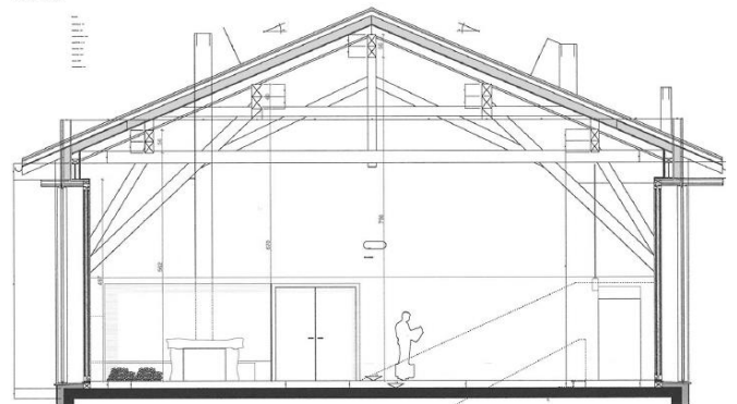
SCHNITTANSICHT A-A Mst. 1:50
